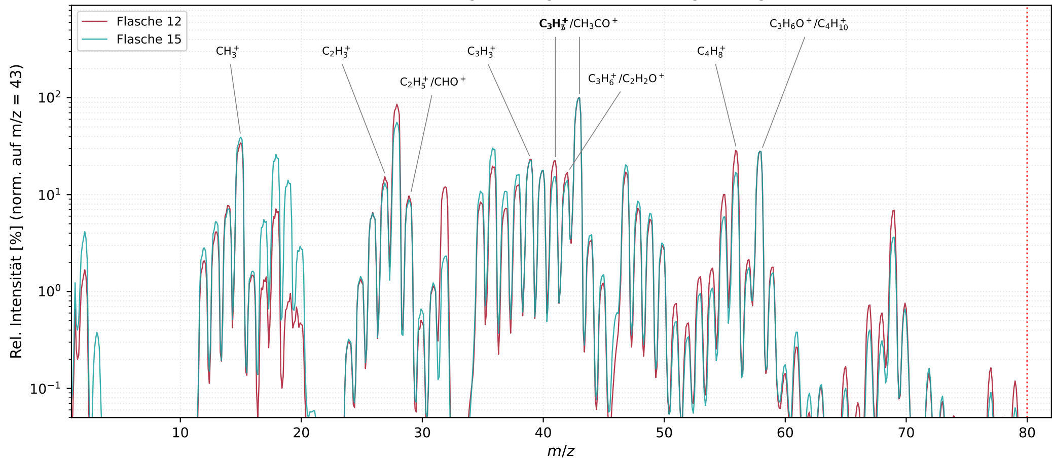
Flasche 12 und 15 - hintergrundkorrigiert, mit Zuordnung der Fragment-Ionen
